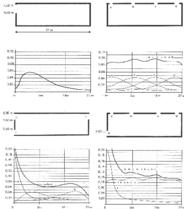
EJEMPLOS de la variación de los E_d sobre el suelo en función de la colocación de las ventanas Trabajo 3
